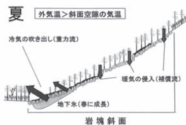
▲図：風穴のしくみ(夏) 【引用】清水長正・澤田結基 編(2015)：日本の風穴、古今書院
